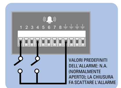
Figura 5. Collegamenti d'allarme
